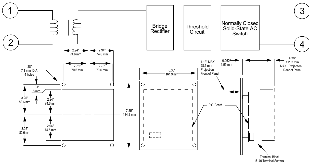
CUTOUT DIMENSIONS
