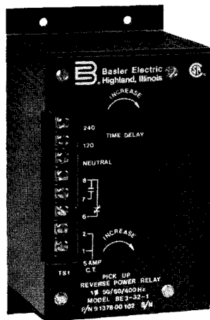
BE3-32-1 (1 Phase)
