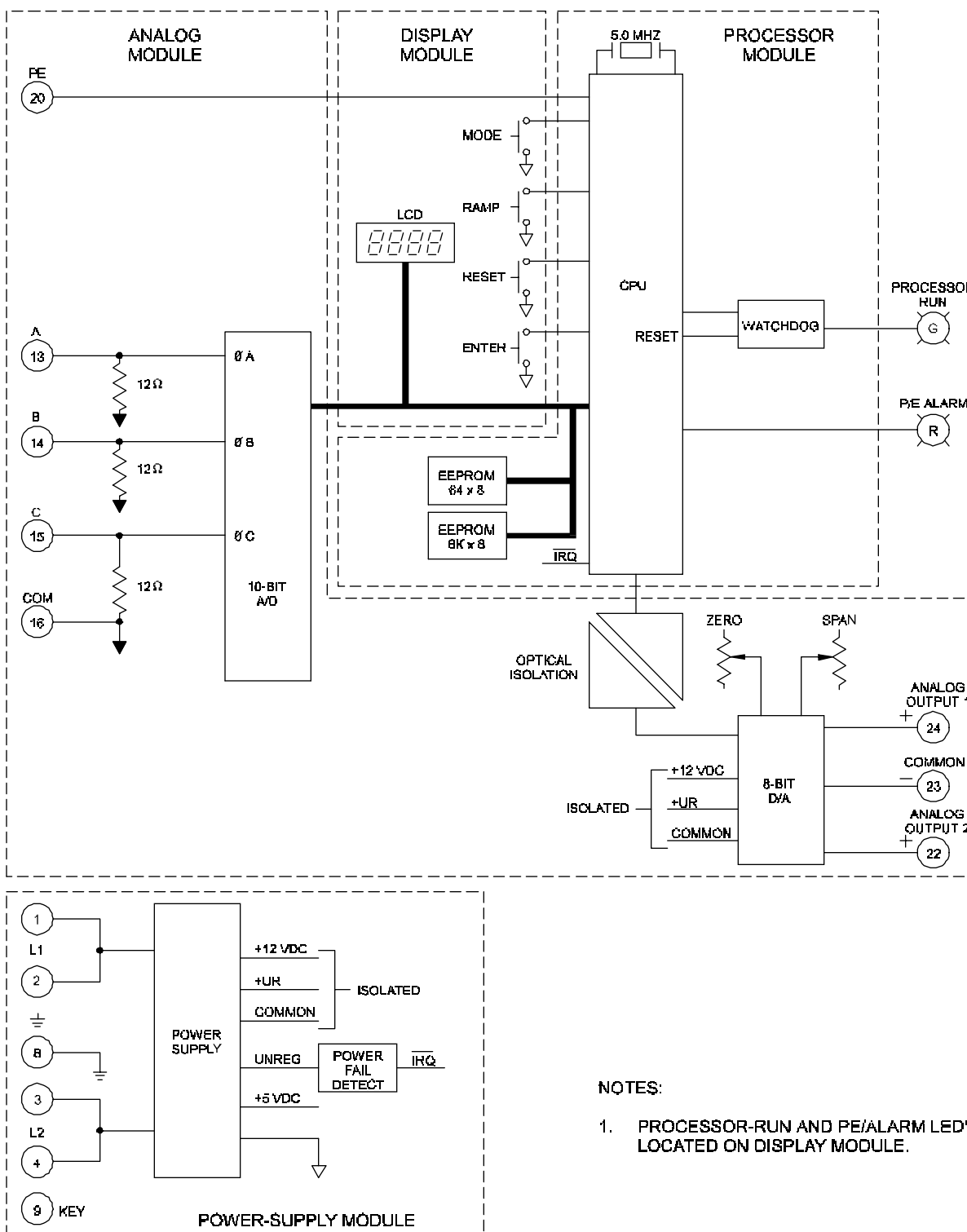
IDM-3 BLOCK DIAGRAM
